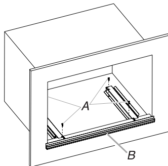
A. Vis à tête cylindrique bombée de 3/4" B. Trousse d'entretoise
