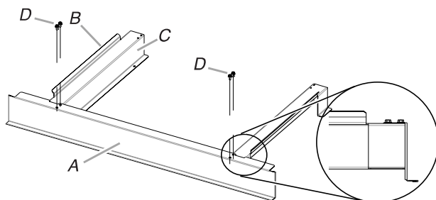
A. Évent inférieur B. Rebord de la barre de calage C. Barres de calage D. Vis rondelle à tête hexagonale de 3/8"
