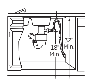
Instalación del eliminador de desechos
