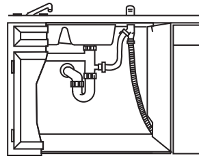
Instalación del eliminador de desechos
