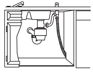
Instalación de la T de desechos
