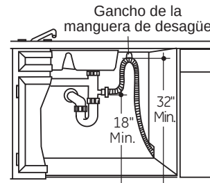
Instalación de la T de desechos
