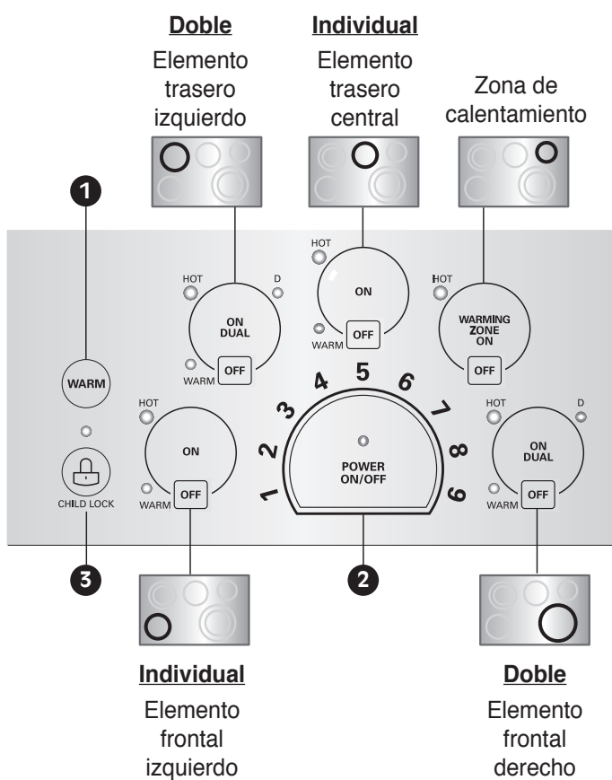
Estufa radiante LSCE305ST
