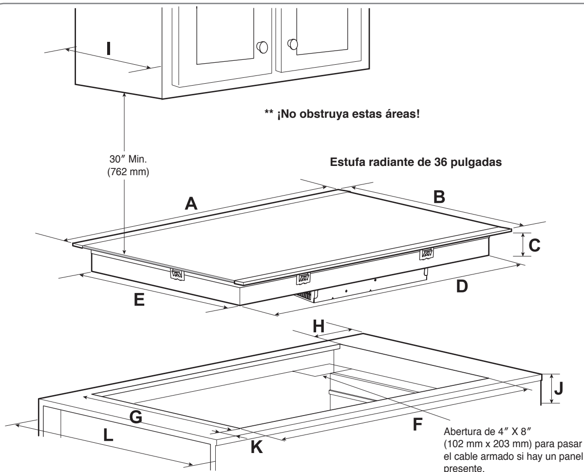
Estufa radiante LSCE365ST
