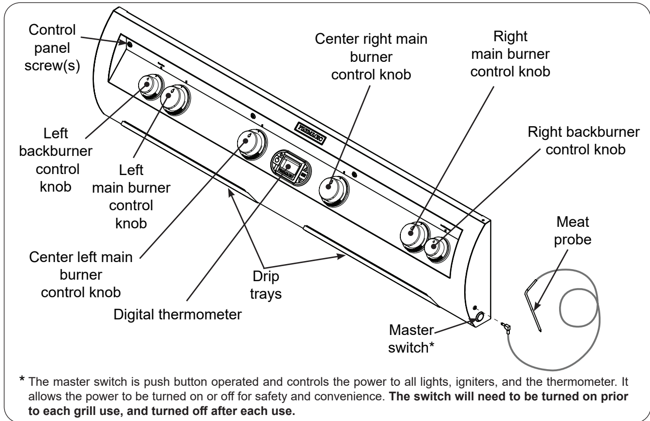
Fig. 27-1 E1060i controls
