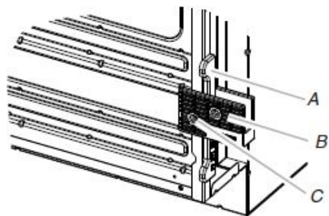
A. Cale B. Pied C. Vis n° 8-18 x 3/8 po (9,5 mm)
