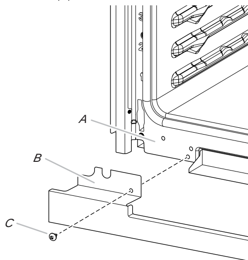
A. Châssis du four B. Onglet de l'évent C. Vis no 8-18 x 3/8 po (9,5 mm)
