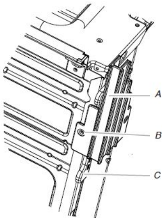
A. Pied avant B. Vis n° 8-18 x 3/8 po (9,5 mm) C. Cale
