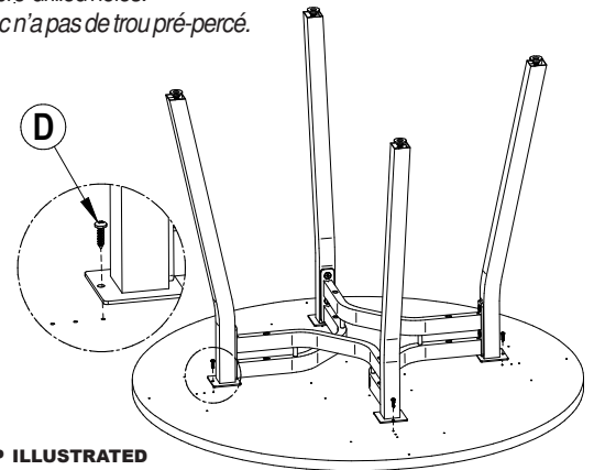
WOOD VENEER TOP ILLUSTRATED DESSUS DE PLACAGE DE BOIS ILLUSTRÉ
