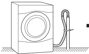
Conexión a la línea de desagüe
