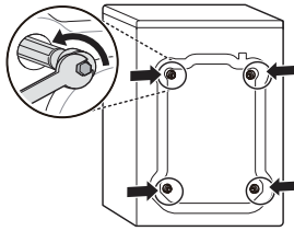
Desembalaje y remoción de los pernos de transporte
