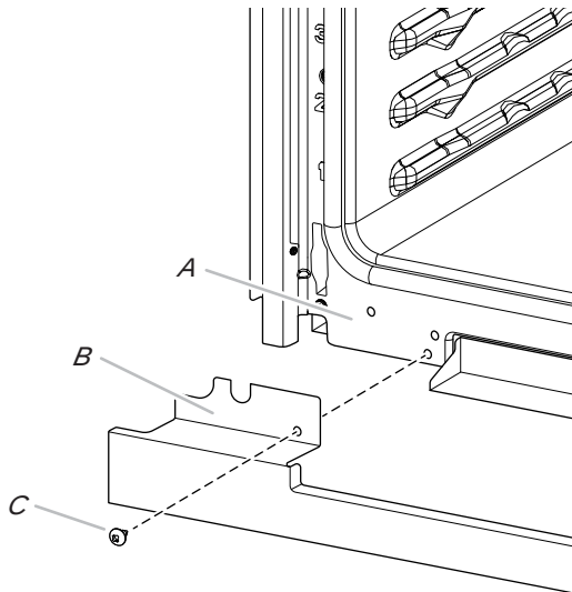
A. Châssis du four B. Onglet de l'évent
