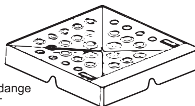
Grille de retour d'air RAVRG2B
