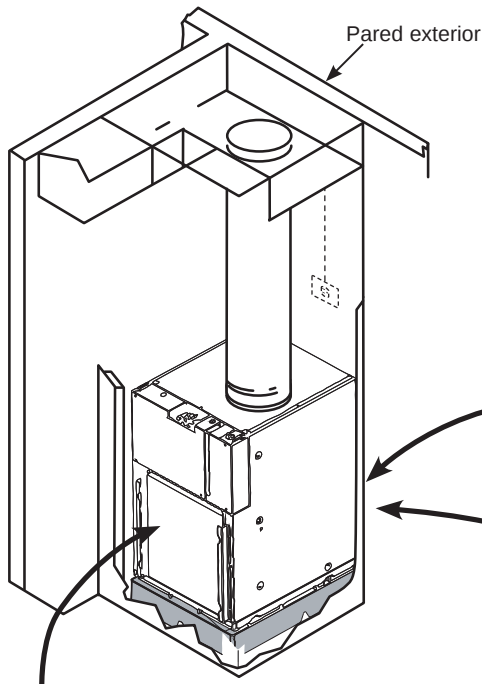
Filtro montado en la unidad con rejilla de retorno de aire suministrada y panel/ puerta de acceso
