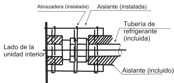
Fig. 4.4 Procedimiento de aislamiento de tuberías
