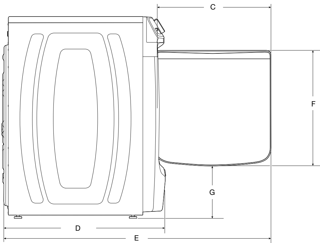
VISTA LATERAL
