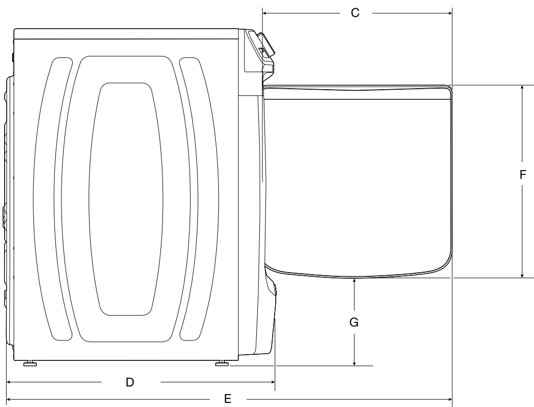
VUE LATÉRALE
