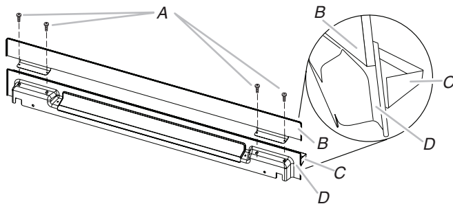
A. Vis n° 8-18 x 1/4" (6,4 mm) B. Déflecteur du tiroir-réchaud C. Évén D. Support de l'évent
