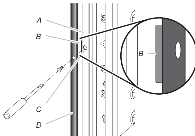
A. Châssis du four B. Espaceur d'installation
