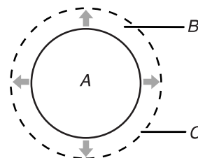
A. Área de cocción de la superficie B. Utensilios de cocina/instrumentos para enlatado C. Saliente máximo de 1/2" (1,3 cm)
